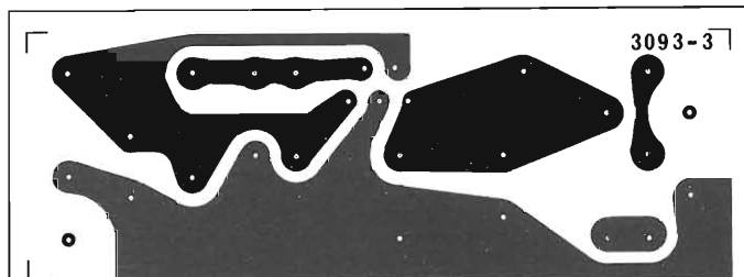
Fig. 2 - Basetta stampata vista dal lato rame in scala naturale. La larghezza delle piste permette senza difficoltà il passaggio di alte correnti.
