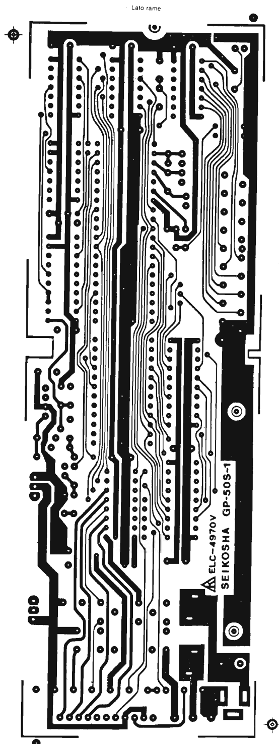
Fig. 4 - Circuito stampato della printer visto dal lato rame e da quello dei componenti leggermente ingrandito. Cortocircuitando il terminale TP a massa, la stampante avvia il ciclo di dimostrazione stampando i caratteri memorizzati in ROM.
