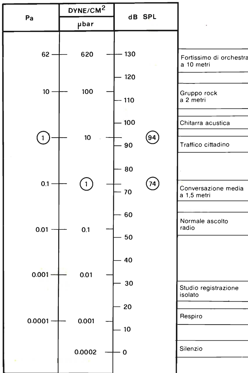
Fig. 1 - Livelli di pressione sonora, all'ingresso del mic, nelle varie unità di misura correnti: Pa, \text{dyne}/\text{cm}^2 , \mu\text{bar} , dB SPL.
